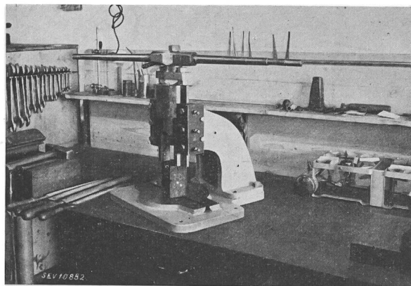
Fig. 11. Elektrisch geschweisste Presse in halbfertigem Zustand
