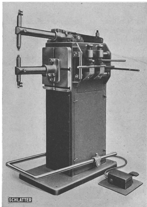
Fig. 17. Punktschweissmaschine bis 50 kVA Seitlich ist Stumpfschweissvorrichtung angebracht
