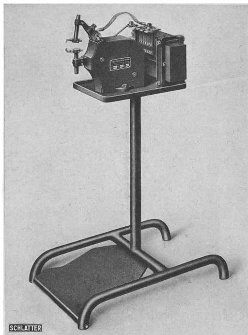
Fig. 16. Kleine Punktschweissmaschine
