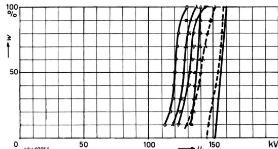
a) 20-kV-Funkenstrecke
