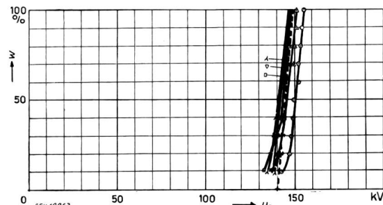
b) 20-kV-Funkenstrecke
