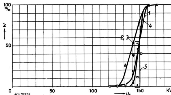
b) 20-kV-Funkenstrecken
