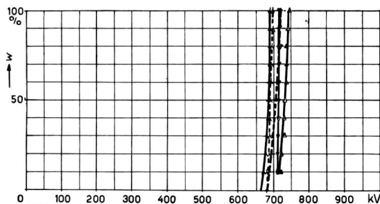
e) 150-kV-Funkenstrecke
