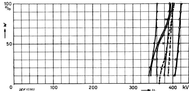
d) 60-kV-Funkenstrecke
