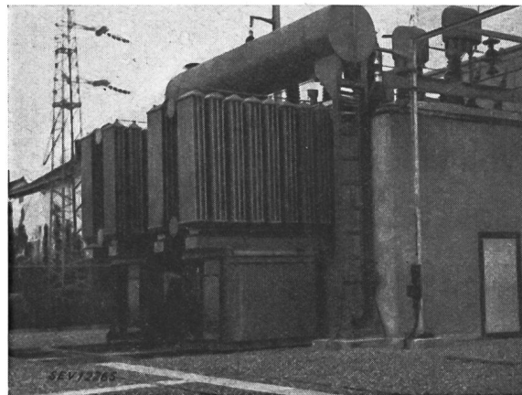
Fig. 7. 35-MVA-Transformator 150/80/50 kV mit natürlichem Oelumlau und forcierter Luftkühlung. Transformator in schalldichter Umbauung. Kühler im Freien.
