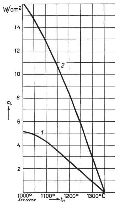
Fig. 3. Oberflächen- belastung p in Funk- tion der Ofentempera- tur t_0 für eine Element- temperatur t_e von 1350° C 1 Element nach Fig. 2. 2 Freistrahler Draht (im Ofen).
