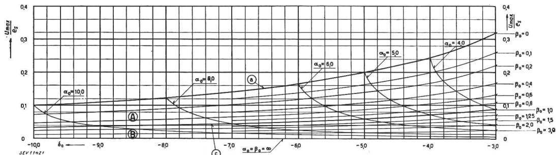
Fig. 6b: Spannungswerte im Abszissenintervall -10 < \epsilon_0 < -3
