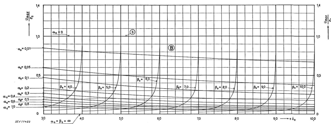
Fig. 6c: Spannungswerte im Abszissenintervall +3 < \epsilon_0 < +10
