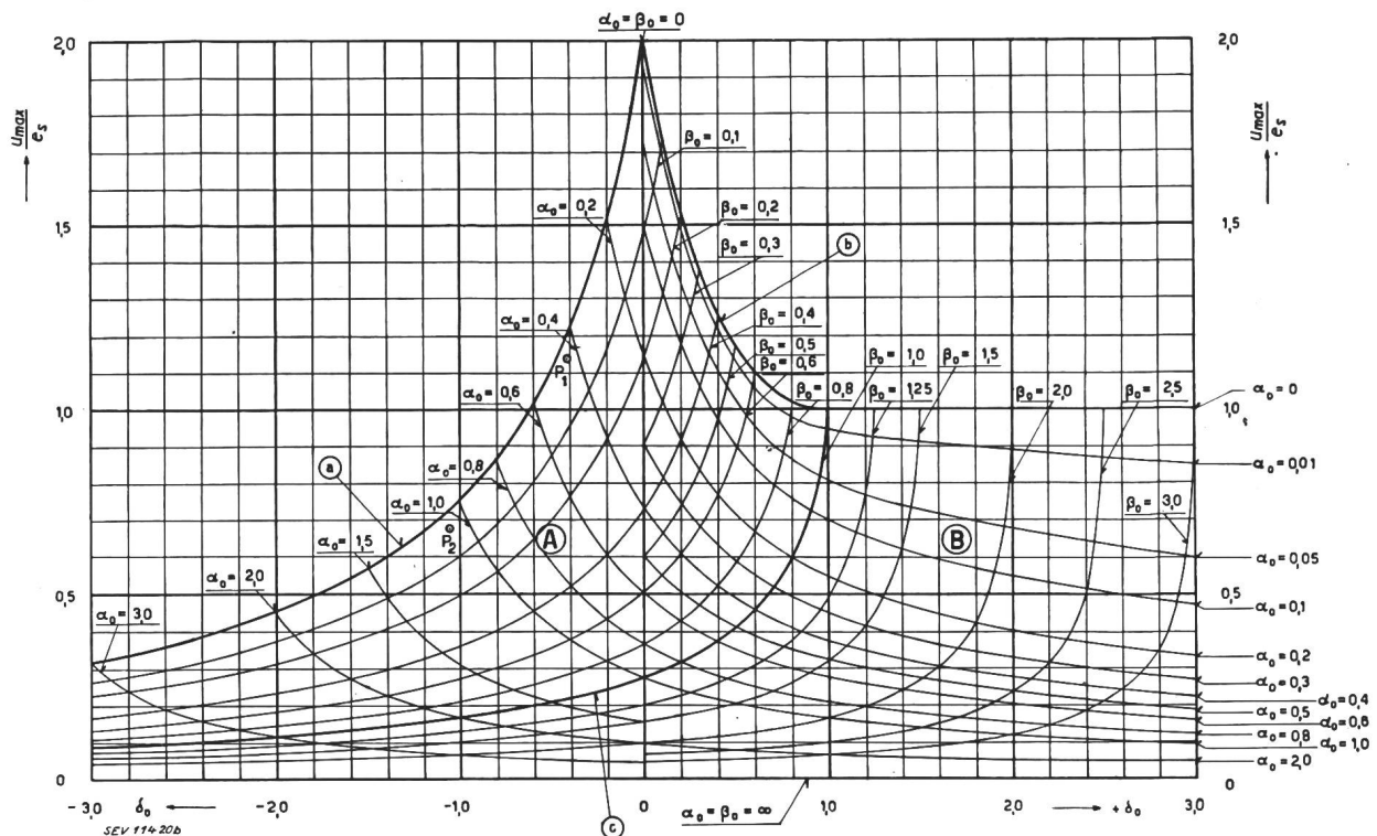
Fig. 6a: Spannungswerte im Abszissenintervall -3 < \epsilon_0 < +3 Spannungsmaximum an der Kapazität in Abhängigkeit von \alpha_0 , \beta_0 und \epsilon_0 .
