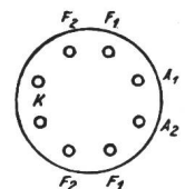
Fig. 7. System und Sockel des Duodiode Der Faden ist aus Symmetriegründen beidseitig herausgeführt.
