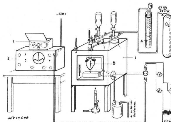
Fig. 2 Versuchsaapparatur
