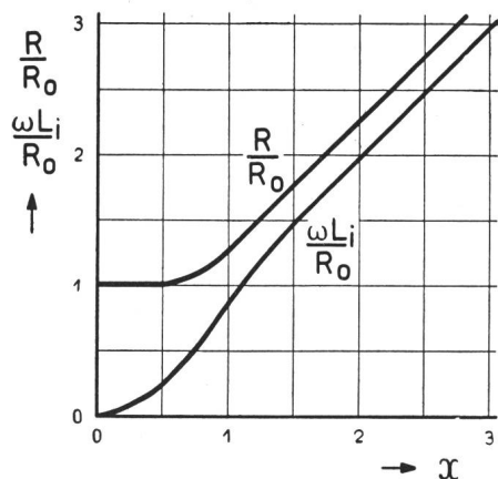
Fig. 5. Skinneffekt am homogenen Runddraht
