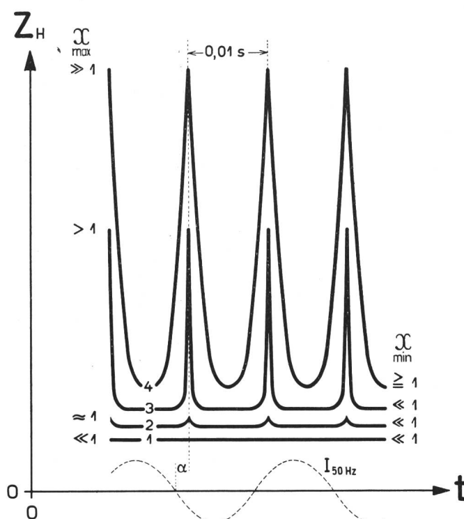
Fig. 7. Typische Pulsationsmuster eines Heizelementes
