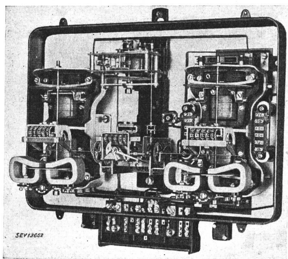
Fig. 2. «Trivector» offen
