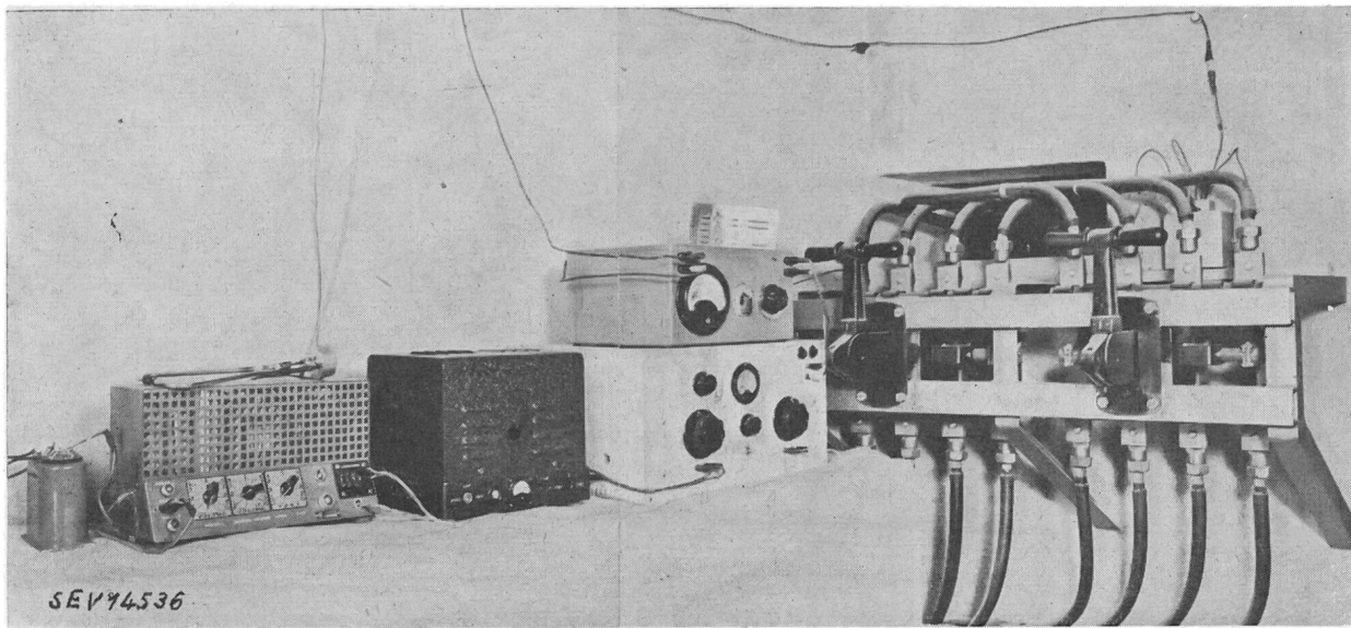
Fig. 1 Netzrundsprich-Versuchsanlage (Airolo)
