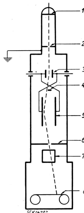
Fig. 1 Vom Verfasser entwickelte Schaltung des Kathodenstrahl- Oszillographen für 40 kV Gleichspannung 1 Kathode 2 Anodenöffnung 3 Ablenkplatten 4 Sperrelektrode 5 Ablenkplatten 6 Schirmplatte 7 Zeitkreisplatte 8 Film
