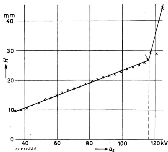
Fig. 6 Graphische Methode zur Fehlerermittlung Auswertung der Oszillogramme für die Phasen V und W des Dreiphasentransformators (siehe Fig. 4). u_s , Stoßspannungs-Scheitelwerte der einzelnen Oszillogrammaufnahmen; H Ordinatenwerte der entsprechenden Stromoszillogramme (ausgemessen in mm) für den Zeitpunkt von 40 μs (nach der Zeitskala). Ergebnis: Beide Wicklungen weisen keinen frühzeitigen Durchschlag auf.
