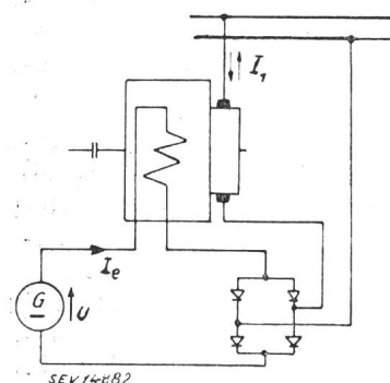
Anwendung der Schaltung zur Speisung der Feldwicklung eines fremderregten Gleichstrommotors
