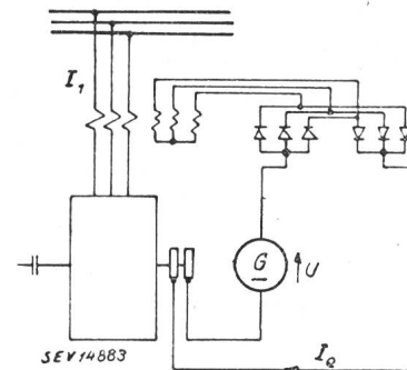
Anwendung der Schaltung zur Erregung eines Synchronmotors (Bezeichnungen wie in Fig. 1)
