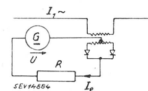
Prinzipschema mit Gleichrichteranordnung in Mittelpunktschaltung
