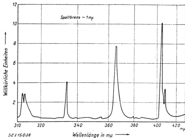
Fig. 8 Spektrale Energieverteilung des Lichtbogens der Quecksilber-Hochdrucklampe HBO 500 im Ultraviolett
