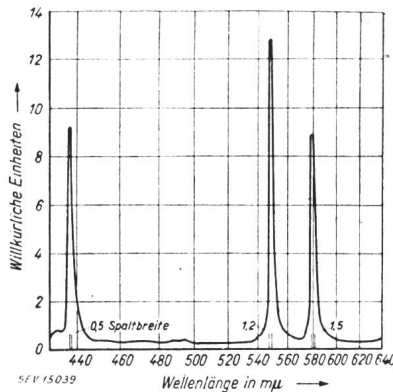
Fig. 9 Spektrale Energieverteilung des Lichtbogens der Quecksilber-Hochdrucklampe HBO 500 im sichtbaren Gebiet
