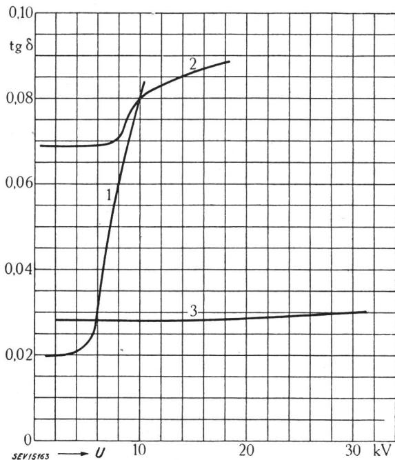
Fig. 9 Spannungsabhängigkeit des Verlustfaktors einiger Nutisolationen
