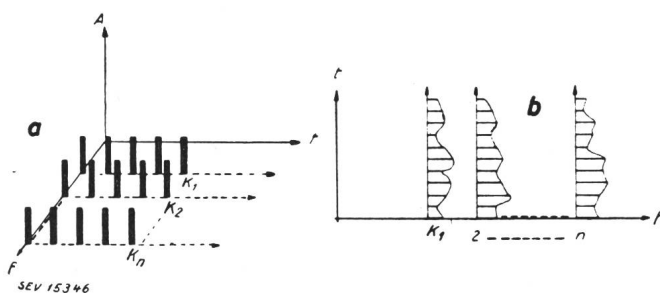
Fig. 5 a Amplitudenmodulation mit vormodulierten Impulsen b Frequenzmodulation mit vormodulierten Impulsen (HF-Amplitude konstant)
