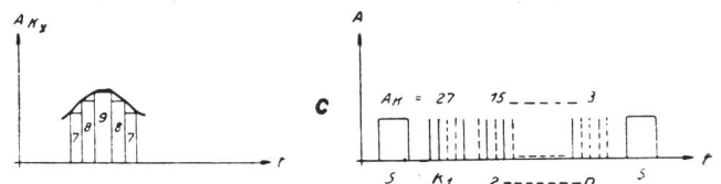
c) Amplitudentastung mit lagemodulierten Impulsen (PTM)
