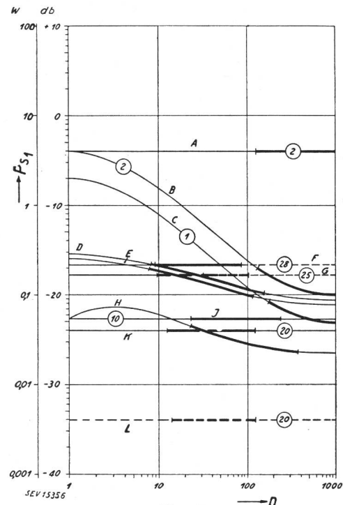
Fig. 15 Erforderliche mittlere Senderleistung pro Kanal mit Rücksicht auf das reine Empfängerrauschen
