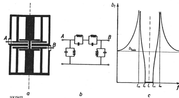
Fig. 10 Topf-Bandfilter a Konstruktion; b Ersatzschema; c Vierpoldämpfung
