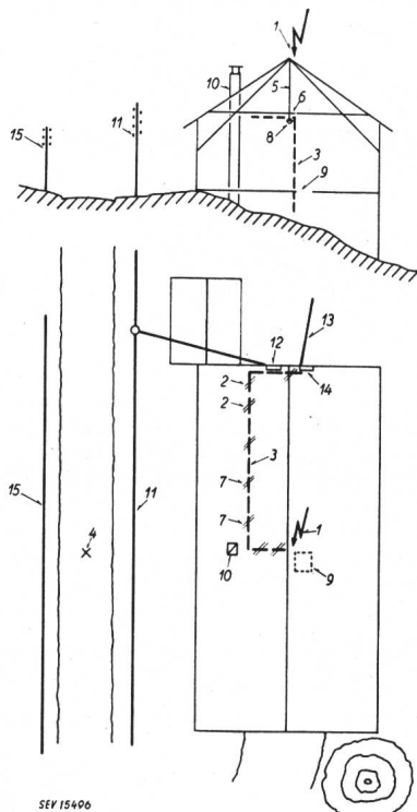
Fig. 1 Lageplan
