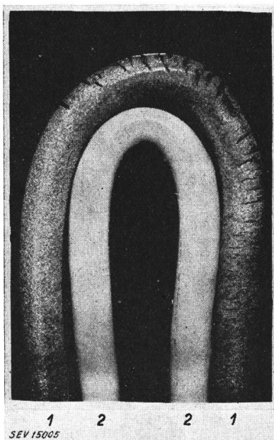
Fig. 5 Câbles isolés exposés 2 heures aux effets d'un mélange air-ozone 1 Caoutchouc naturel 2 Thermoplaste à base de chlorure de polyvinyle
