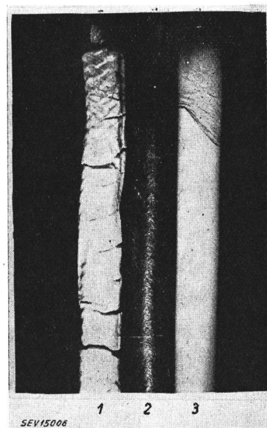
Fig. 6 Câbles isolés immergés 4 jours dans l'huile puis étuvés 4 jours à 80 °C 1 Caoutchouc naturel 2 Caoutchouc synthétique (Néoprène) 3 Thermoplaste à base de chlorure de polyvinyle
