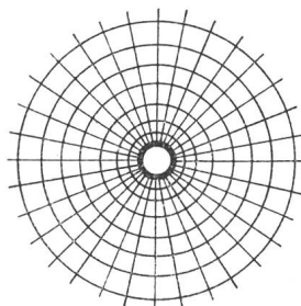
Hohlseil Verminderte Feldstärke am Leiterumfang, verringertes Sprühen
