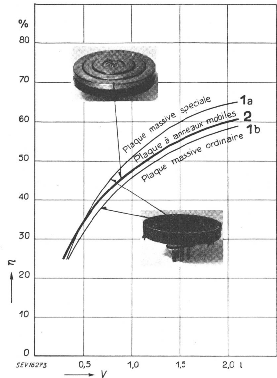
Fig. 5 Rendement «à froid» en % (voir Règles ASE) en fonction du volume d'eau chauffé, V en litres
