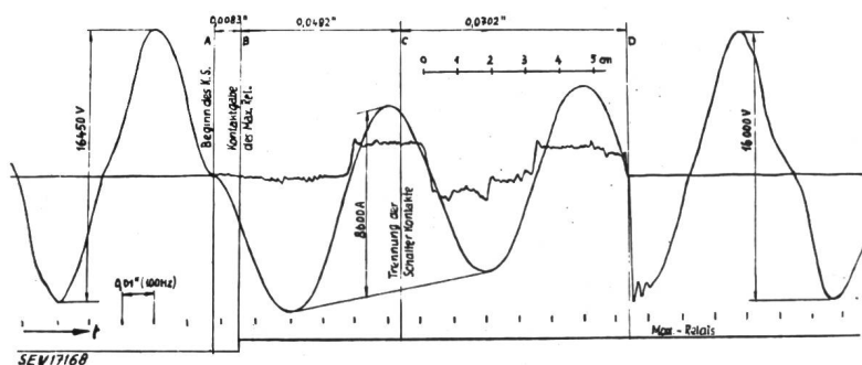
Fig. 4 Oszillogramm der Abschaltung eines Kurzschluss- stromes von 8600 A bei 16 kV durch den Öl- strahlschalter HPF 7 - 16 2 / 3 Hz (Nennspannung 30 kV, Nennstrom 1000 A, Nenn- ausschaltleistung 250 MVA bei 16 kV) Aufgenommen anlässlich der Abschaltversuche im Unterwerk Seebach der SBB A Beginn des Kurzschlussstromes; B Kontaktgabe des Maximal-Relais; C Trennung der Schalter- kontakte; D Löschpunkt des Lichtbogens
