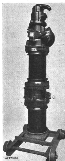
Fig. 5 Ölstrahlschalter HP 7 - 16 2 / 3 Hz für Innenraumaufstellung (Nennspannung 20 kV, Nennstrom 1000 A, Nennausschaltleistung 250 MVA bei 16 kV) Eingebaut als Fahrleitungs-Speise- punktschalter im Netz der SBB
