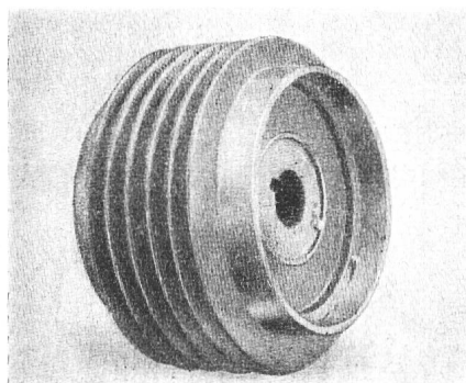
Fig. 10 Keilriemen-Kupplung
