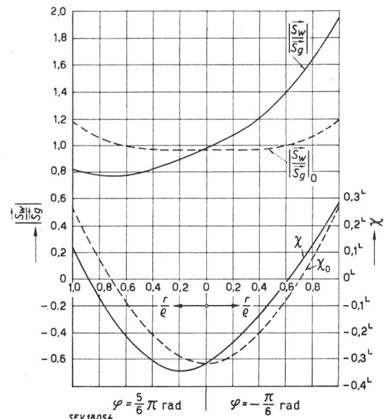
Fig. 4 Verlauf der Stromdichte im Leiter 1 nach Betrag und Phasenwinkel für einen bestimmten Durchmesser — mit Nähwirkung --- ohne Nähwirkung
