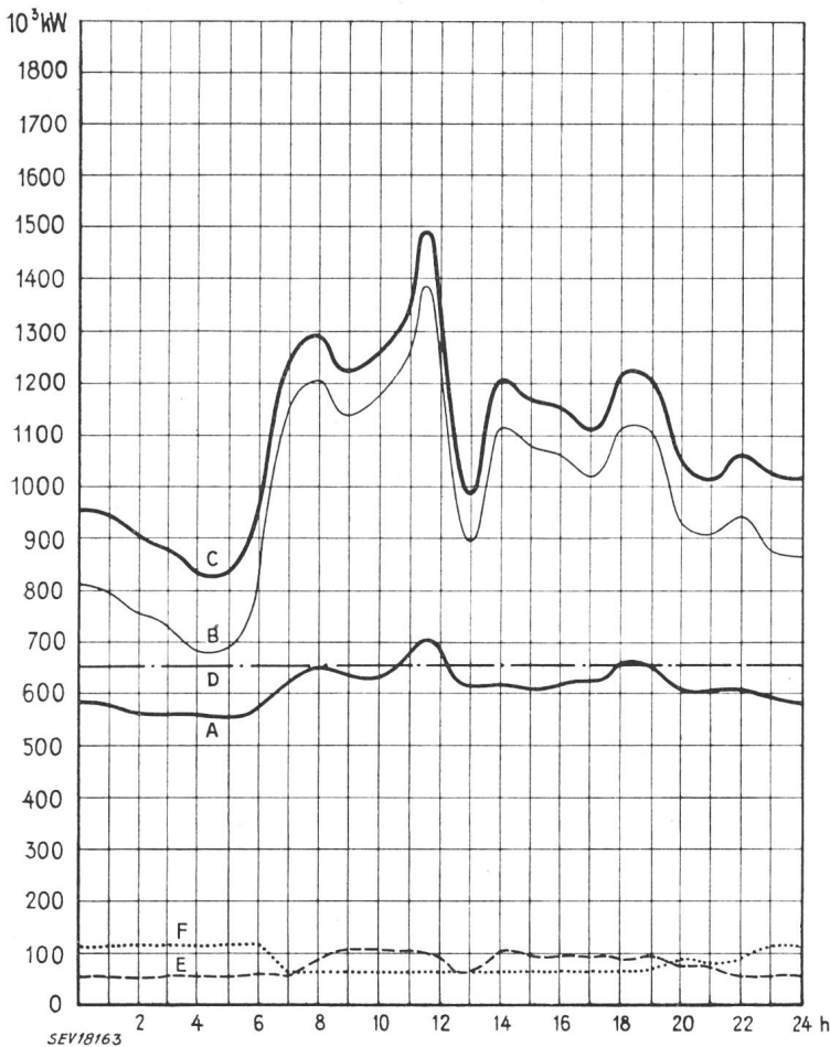
Tagesdiagramme der beanspruchten Leistungen. Mittwoch, 14. Februar 1951
