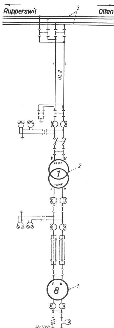
Fig. 2 Kraftwerk Gösgen, Einphasen-Anlage 16 \frac{2}{3} Hz 1 Generator 12 000 kVA, 10,5 kV 2 Transformator 12 000 kVA 3 66-kV-Übertragungsleitungen der SBB
