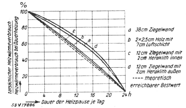
Fig. 7 Mögliche Ersparnisse an Heizwärme bei unterbrochener Heizung gegenüber Dauerheizung bei 0 bis 24 h täglicher Heizpause
