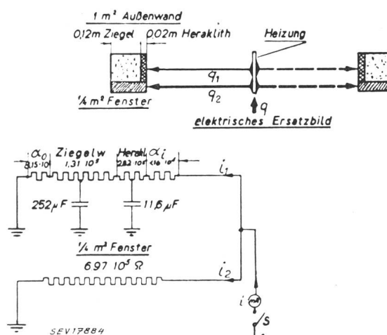
c) Ziegelwand mit Heraklith-Innenauskleidung
