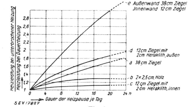
Fig. 8 Erforderliche Erhöhung der Heizleistung bei unterbrochener Heizung gegenüber Dauerheizung bei 0 bis 24 h täglicher Heizpause
