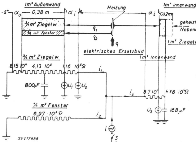
Fig. 9 Bauliche Anordnung und Modellbild für den Fall e t_1 Temperatur der inneren Oberfläche der Aussenwand entsprechend der Spannung U_1 t_2 Temperatur der inneren Oberfläche der Innenwand entsprechend der Spannung U_2 Weitere Bezeichnungen siehe Fig. 5
