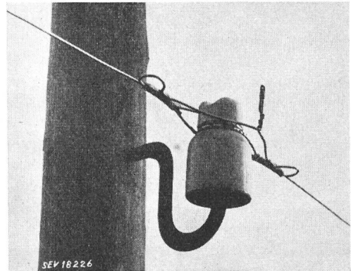
Fig. 5 Fertig geschweisste Verbindung
