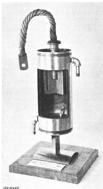
Fig. 1 Ignitron Schalterröhre Maximale Schaltleistung 1200 kVA
