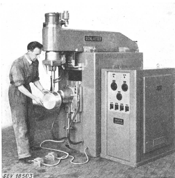
Fig. 16 Kombinierte 3-Phasen-Punkt- und Nahtschweissmaschine Maximalleistung 300 kVA
