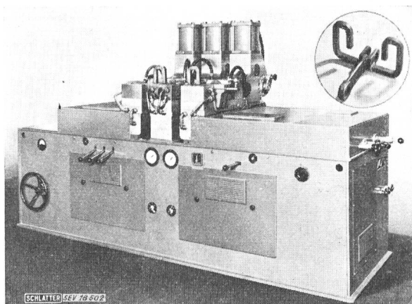
Fig. 15 Doppeltwirkende Abschmelzschweissmaschine, gespeist durch ein 3-Phasen-Lastausgleichgerät
