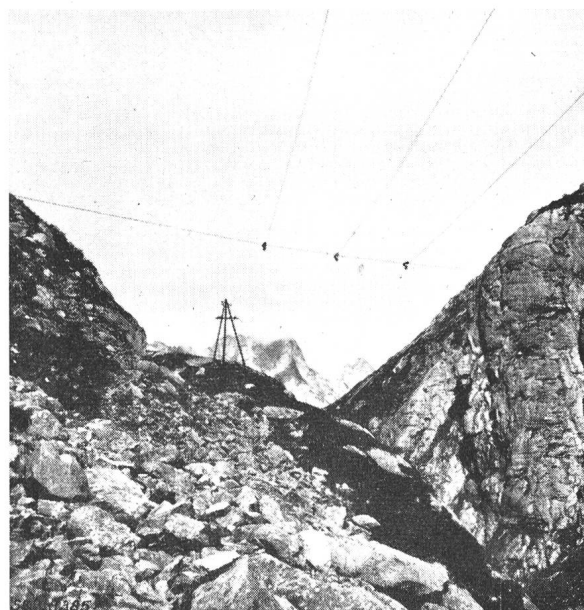
Fig. 5 Queraufhängung
