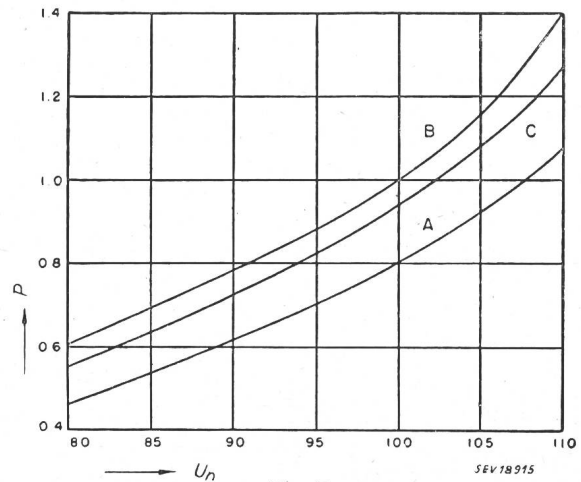
Fig. 7 Eisenkernverluste in Funktion der angelegten Netzspannung in %
