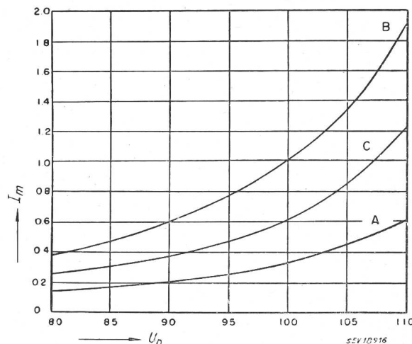
Fig. 8 Magnetisierungsstrom in Funktion der angelegten Netzspannung in %
