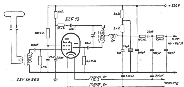
Fig. 6 UKW-Pendelrückkopplungs-Empfänger
