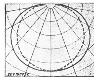
Strahlungsverteilung in den zwei Hauptachsen
