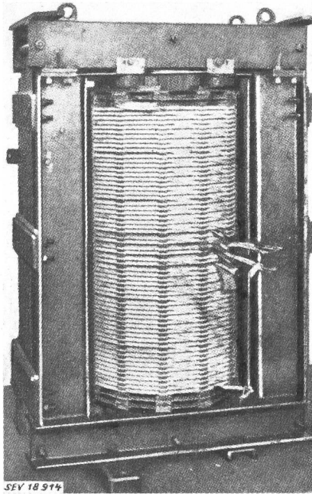
Fig. 6 Zusammengebauter Wickelkern-Transformator
