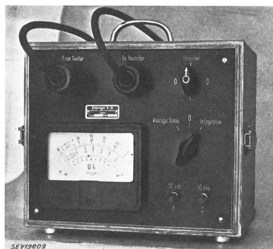
Fig. 9 Integrator zur Bestimmung der mittleren Ungleichmässigkeit eines Querschnittsverlaufes
