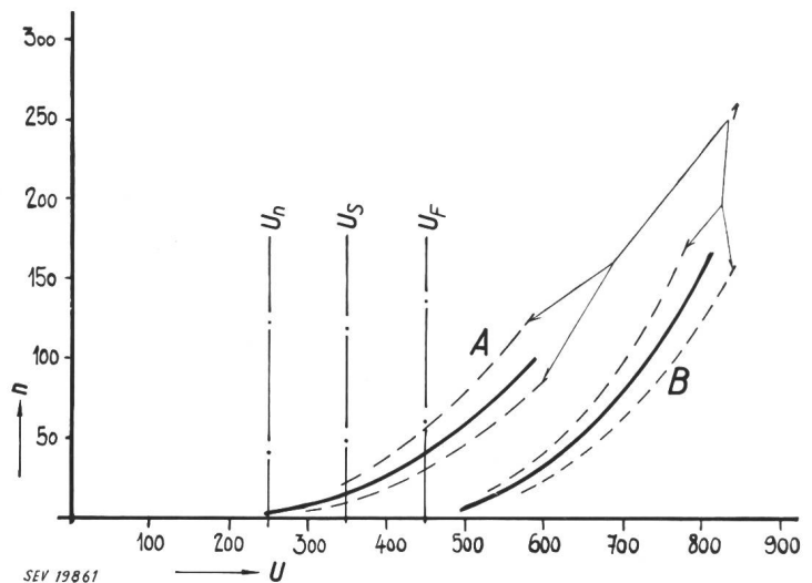
Fig. 8 Zahl der Durchschläge in Abhängigkeit der an den Kondensator angelegten Gleichspannung A 1. Versuch { mit derselben Serie; Kondensatoren des Typs WMH, 1 \mu F, 250/350 V— und 110/160 V~ (Condensateurs Fribourg) B 2. Versuch { n Zahl der Durchschläge; U Spannung; I Streugebiet
