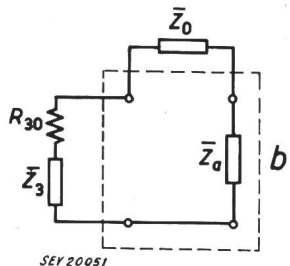
Fig. 9 Impédances négatives connectées à un circuit d'impédance \bar{Z}_0 a Impédance négative-parallèle b Impédance négative-série Mêmes notations que dans fig. 6 à 8
