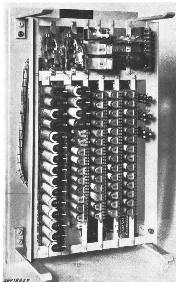
Fig. 3 Fernsteuer-Wählerapparat für Wandschrank
