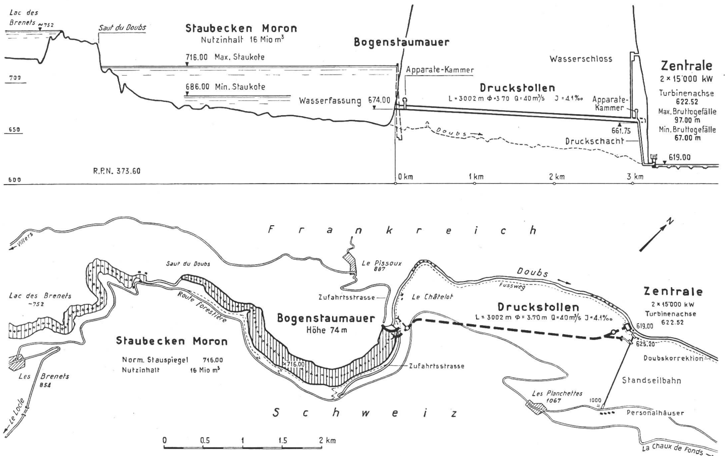
Fig. 2 Lageplan und Längenprofil 1 : 50 000
