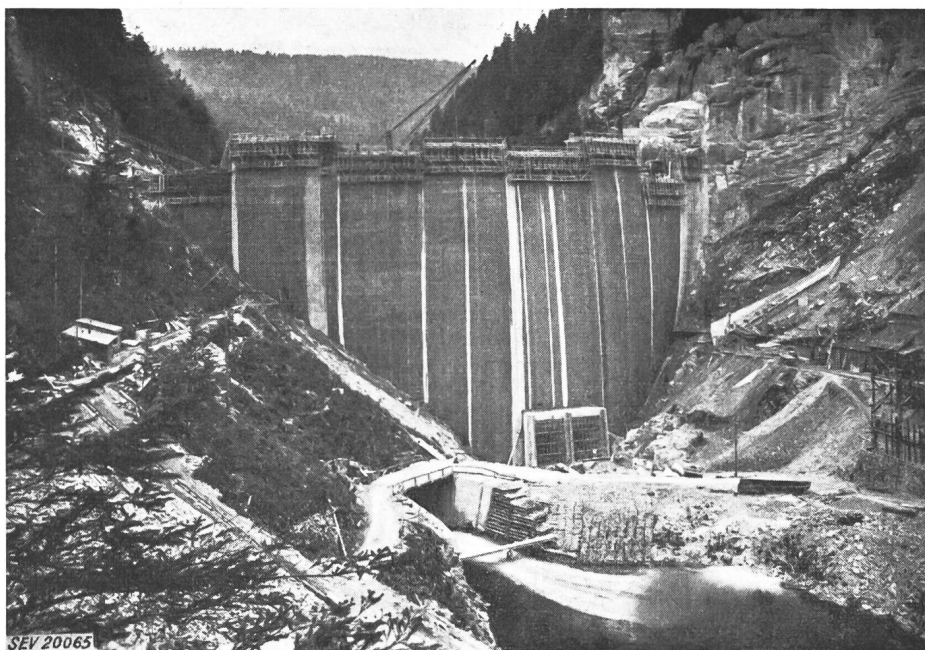
Fig. 6 Staumauer Ansicht von der Wasserseite Bauzustand Juni 1952
