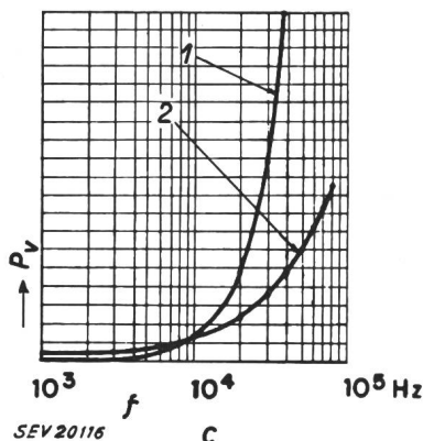
Fig. 6 Erklärung der Hysteresisverluste
