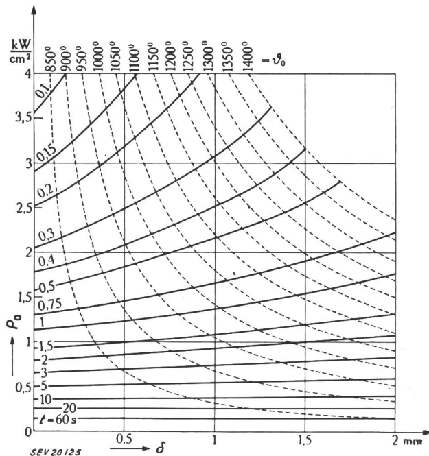
Fig. 15 Härteprofil \delta in Funktion der Oberflächenleistung P_0 \delta Härtetiefe in mm P_0 Oberflächenleistung in kW/cm 2 Parameter: t Zeit in s; \vartheta_0 Temperatur in °C
