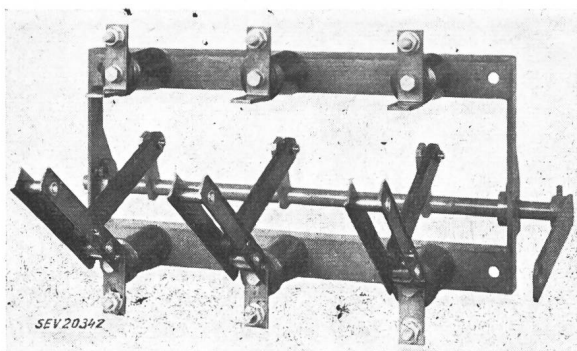
Fig. 1 Einfacher Trenner
