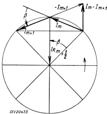
Fig. 2 Darstellung der verschiedenen Ströme im Käfiganker
