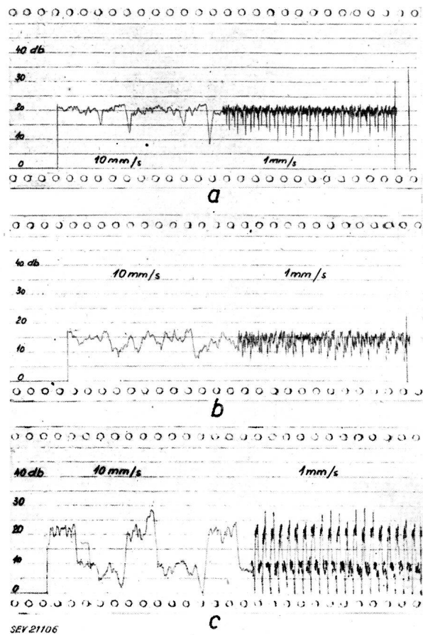
Fig. 6 Störspannung am Ausgang eines Radioempfängers, hervorgerufen durch eine Leuchtstoffröhre a Abstimmfrequenz des Empfängers 550 kHz; b Abstimmfrequenz des Empfängers 1 MHz; c Abstimmfrequenz des Empfängers 1,4 MHz
