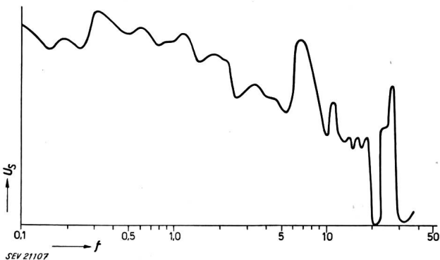
Fig. 7 Qualitativer Verlauf der Störspannung am Ausgang eines Radioempfängers, hervorgerufen durch eine Leuchtstofflampe, in Funktion der Eingangsspannung Us niederfrequente Störspannung; f Abstimmfrequenz des Empfängers (MHz)
