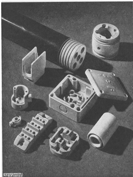
Fig. 4 Steatit-Teile
