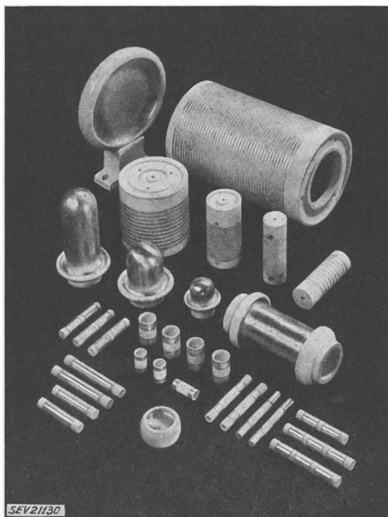
Fig. 6 Kondensatoren
