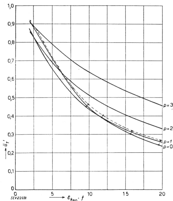
Fig. 8 Spannungsverhältnis \ddot{u}_T' = U_1'/U_1 eines Transformators in Funktion der Frequenz f in kHz und der relativen Kurzschluss-Spannung \varepsilon_{k50} bei 50 Hz in %
