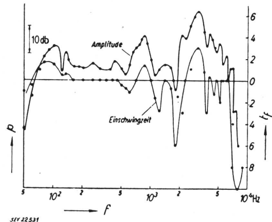
Fig. 1 Amplitudenkurve und Einschwingkurve eines elektrodynamischen Lautsprechers nach Helmholtz p Schalldruck; f Frequenz; t_f Einschwingzeit in Periodenzahl
