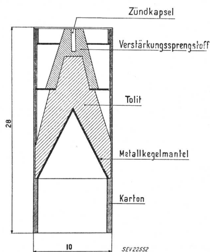
Fig. 2 Schematischer Querschnitt einer Ladung
