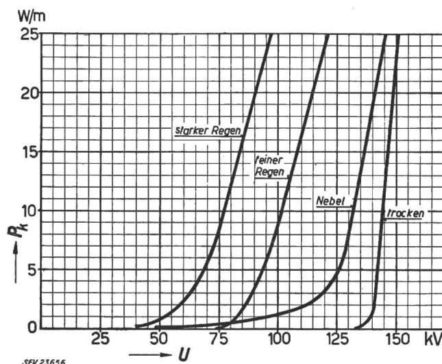
Fig. 1 Koronaverluste P_k eines Al-Seiles mit Runddrahtdecklage von 26 mm Durchmesser bei verschiedenen Witterungsbedingungen in Abhängigkeit von der Versuchsspannung U in der Reuse Barometerstand b = 730 mm Hg; Temperatur t = 20^\circ\text{C}
