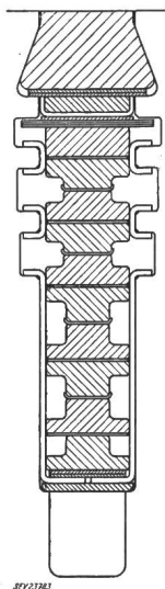
Fig. 24 Rotornuten von BBC-Turbomaschinen mit Wasserstoffkühlung
