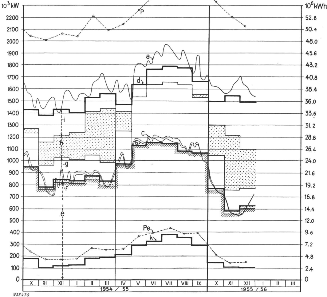
Mittwoch- und Monatserzeugung der Elektrizitäts- werke der Allgemeinversorgung
