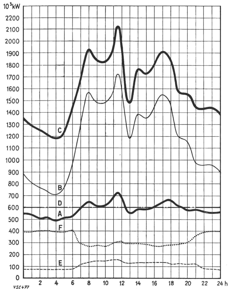
Tagesdiagramme der beanspruchten Leistungen (Elektrizitätswerke der Allgemeinversorgung) Mittwoch, den 14. Dezember 1955
