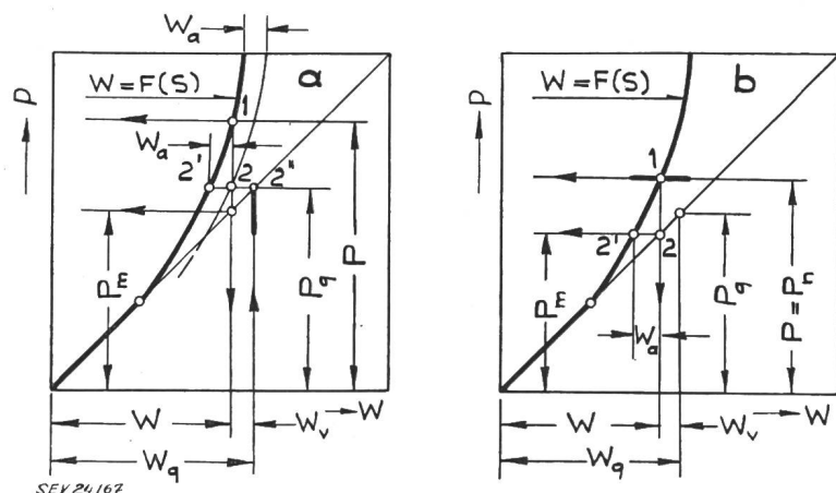
Fig. 4 Beschränkungen in der Ausnutzung der naturbedingt anfallenden Energiemengen W_q a vom Energiespeicher W_q ; b von der installierten Leistung P_n
