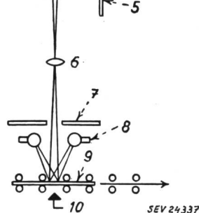
Fig. 1 Optisches System zum Lesen einer Textzeile
